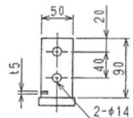
一次端子詳細図
