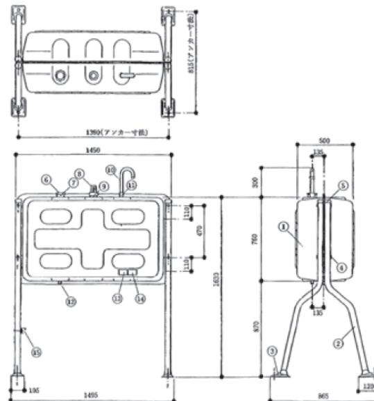
HT-K490型ダイケンホームタンク 角形
