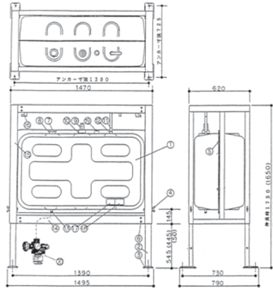
RTS-K490JU レンタルタンク
